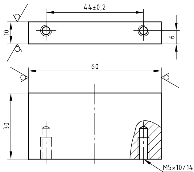
Skizze 2 \sqrt{Rz\ 16} ( \checkmark )
