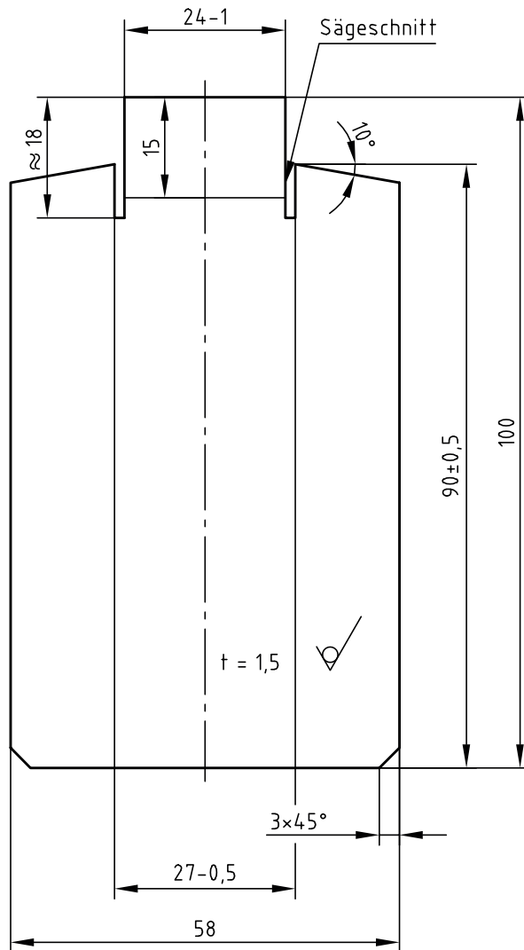
Skizze 7 \sqrt{Rz\ 16} ( \checkmark )
