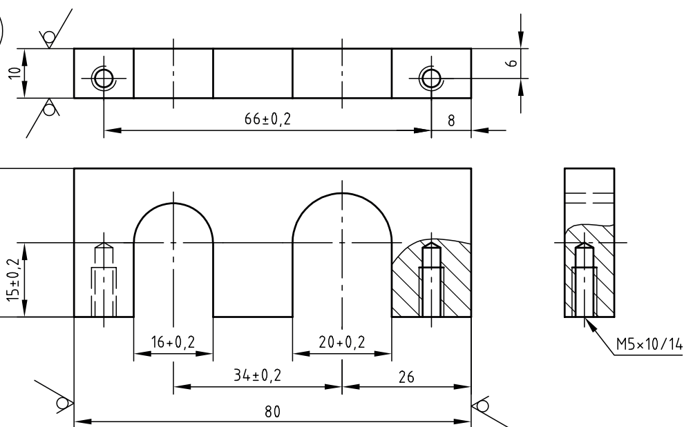
Skizze 3 \sqrt{Rz\ 16} ( \checkmark )
