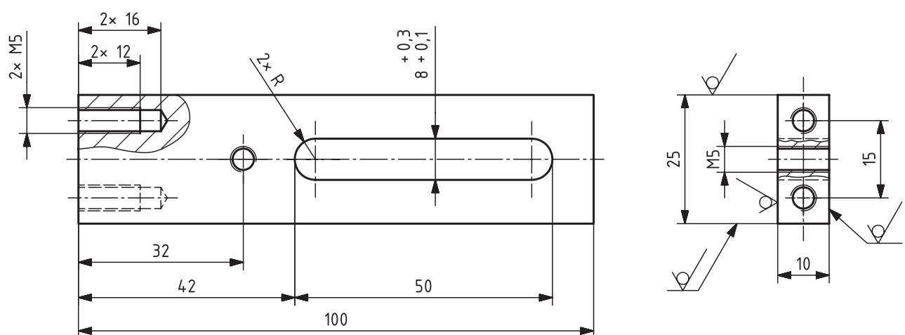
Skizze 4 \sqrt{Rz\ 16} (✓)
