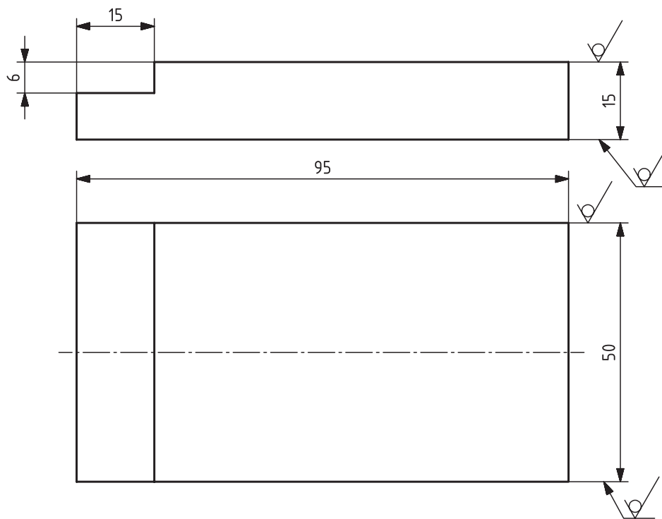
Skizze 4 \sqrt{Rz\ 16} (✓)
