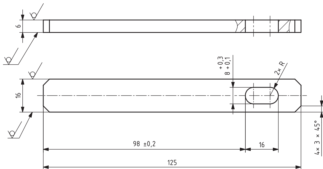
Skizze 8 \sqrt{Rz\ 16} (✓)
