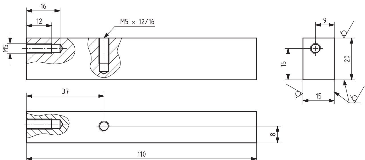
Skizze 5 \sqrt{Rz\ 16} (✓)
