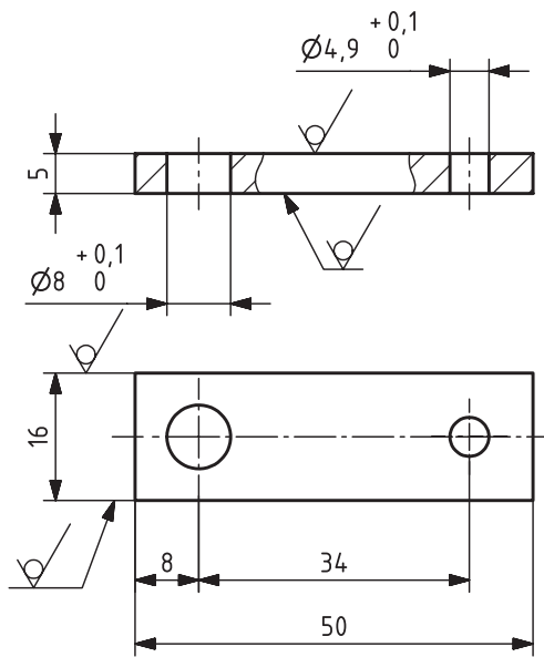
Skizze 9 \sqrt{Rz\ 16} (✓)
