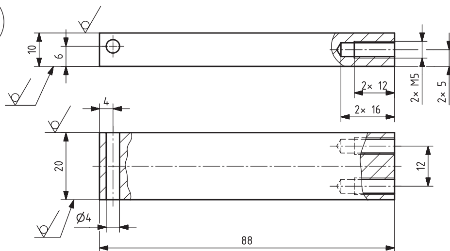
Skizze 7 \sqrt{Rz\ 16} (✓)
