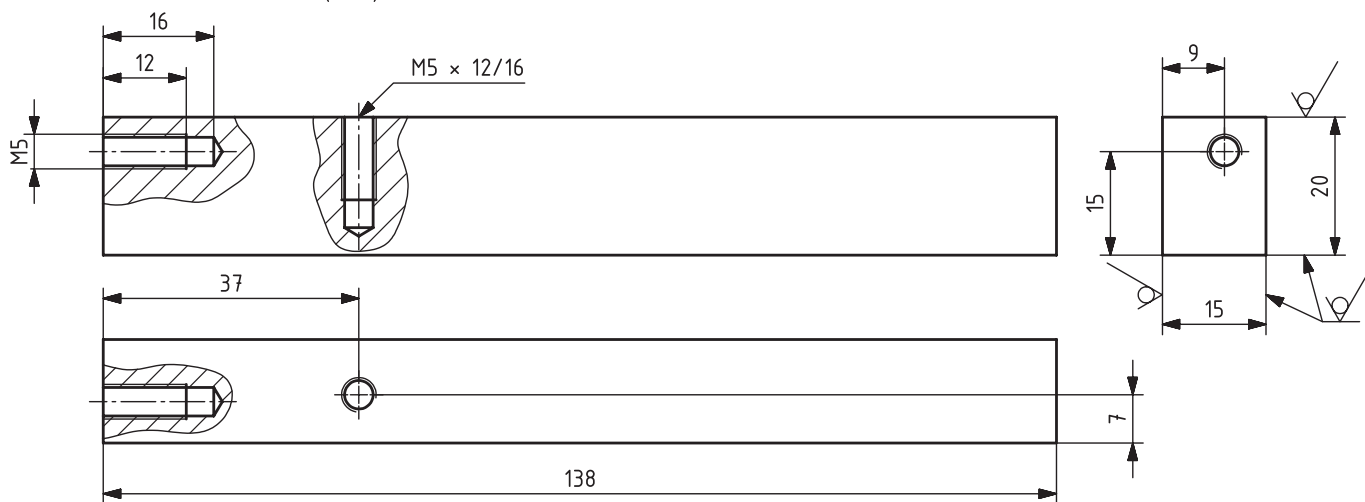
Skizze 7 \sqrt{Rz\ 16} (✓)
