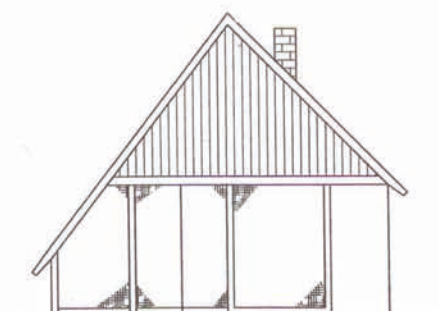
Ansicht Süd
