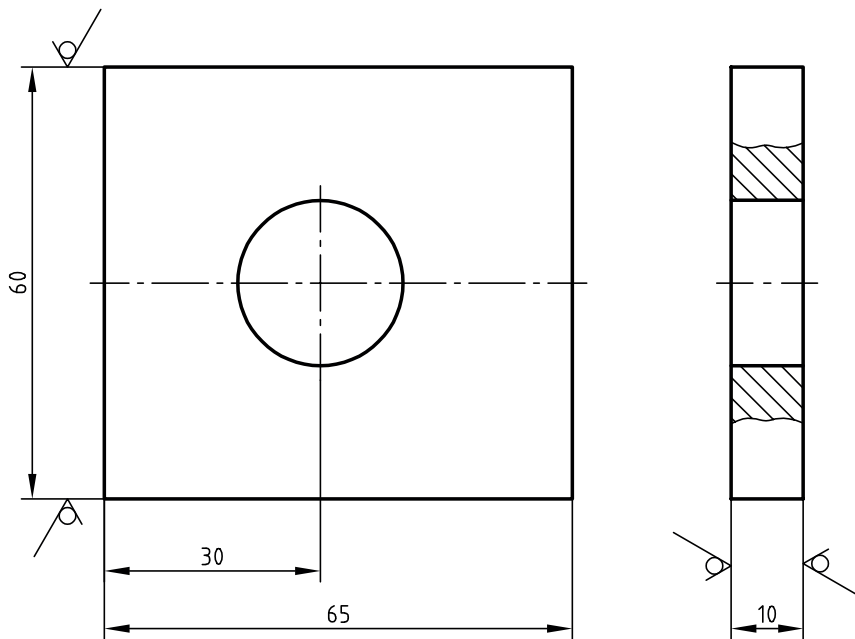
Skizze 1 \sqrt{Rz\ 16} ( \checkmark )
