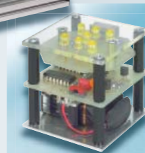
Projektarbeit „Elektronischer Würfel“
