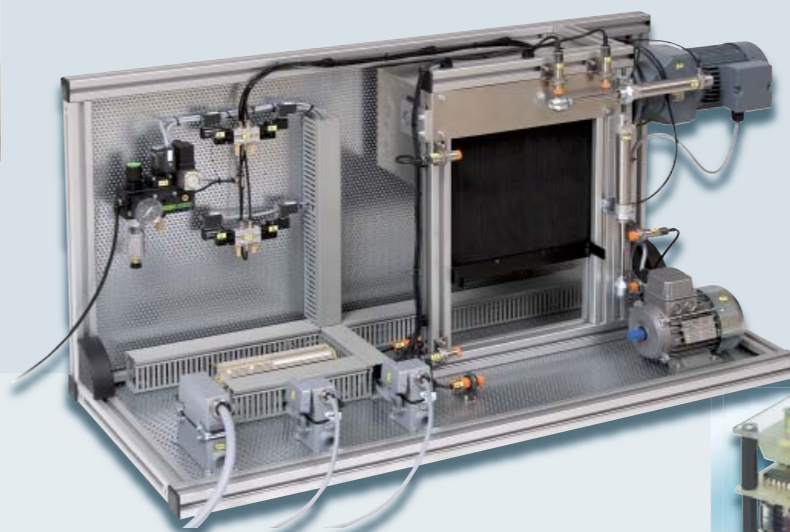
Projektarbeit „Rolltor“, eine Entwicklung der Volkswagen Coaching GmbH
